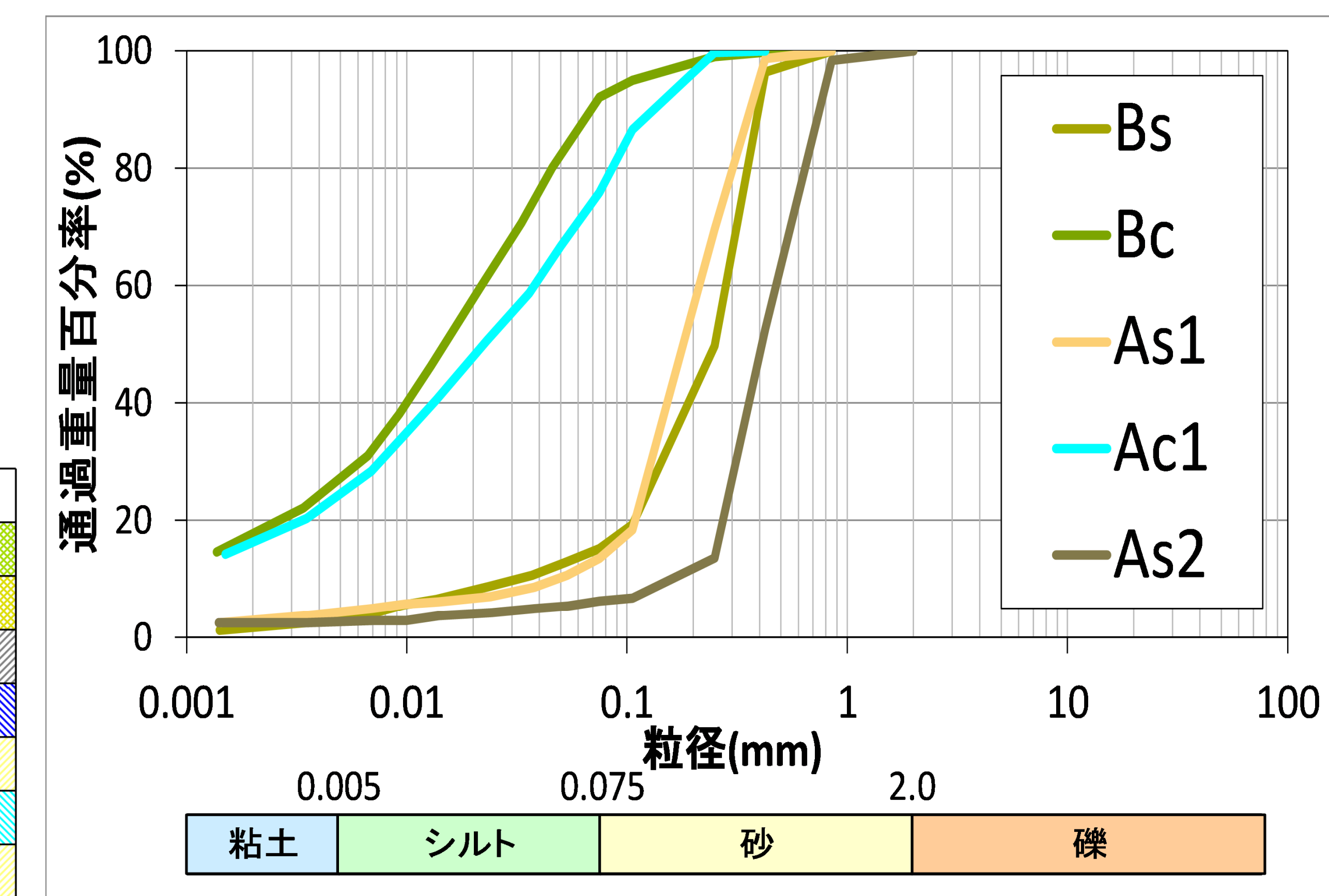
粒径加積曲線図
