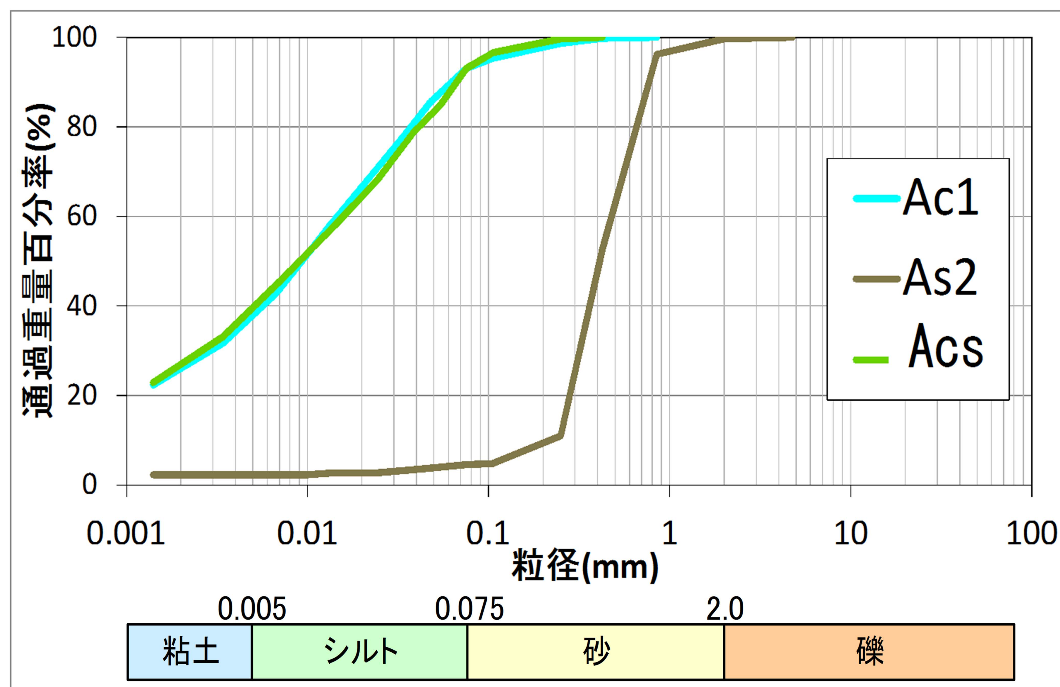
粒径加積曲線図
