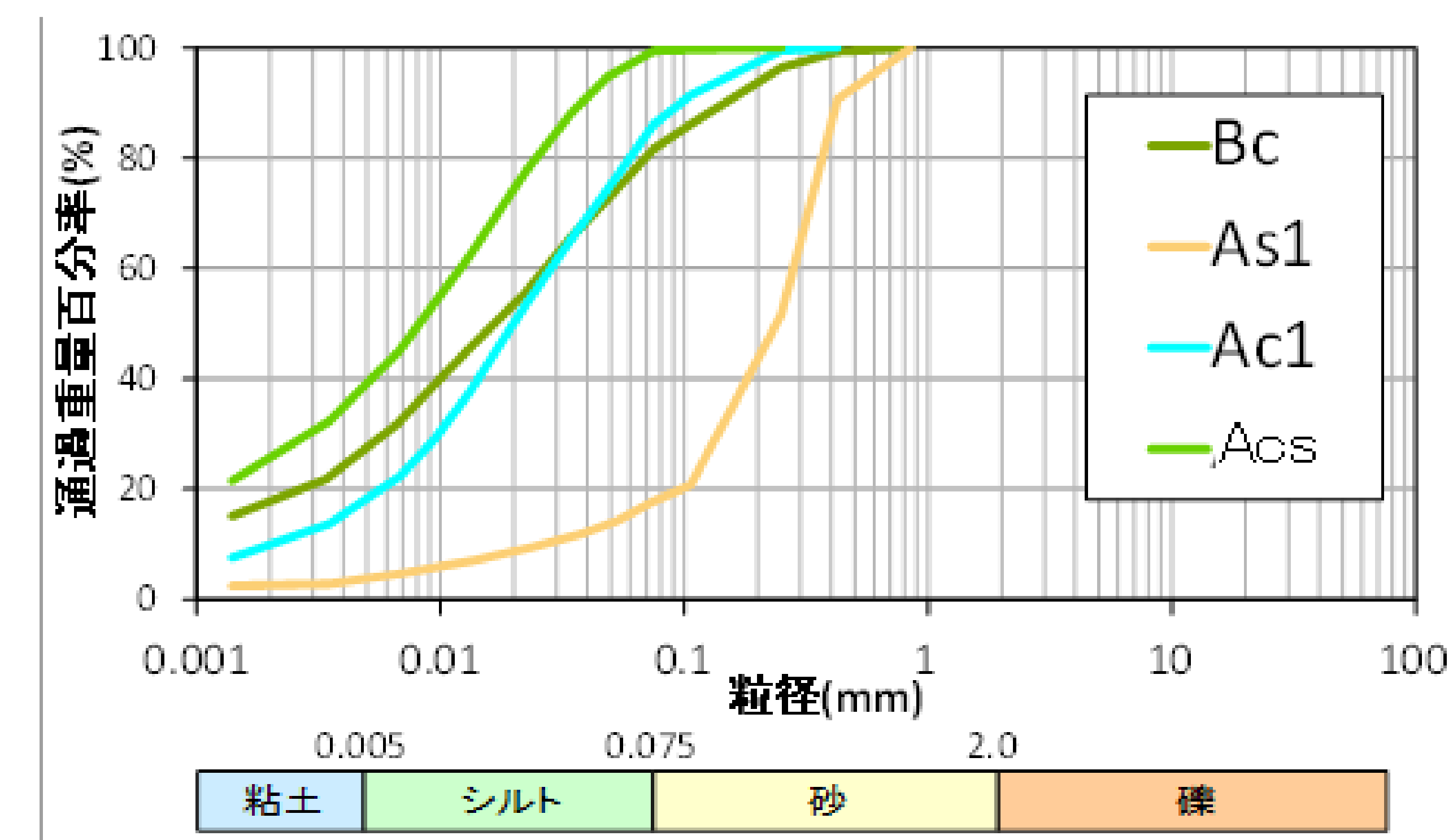
粒径加積曲線図
